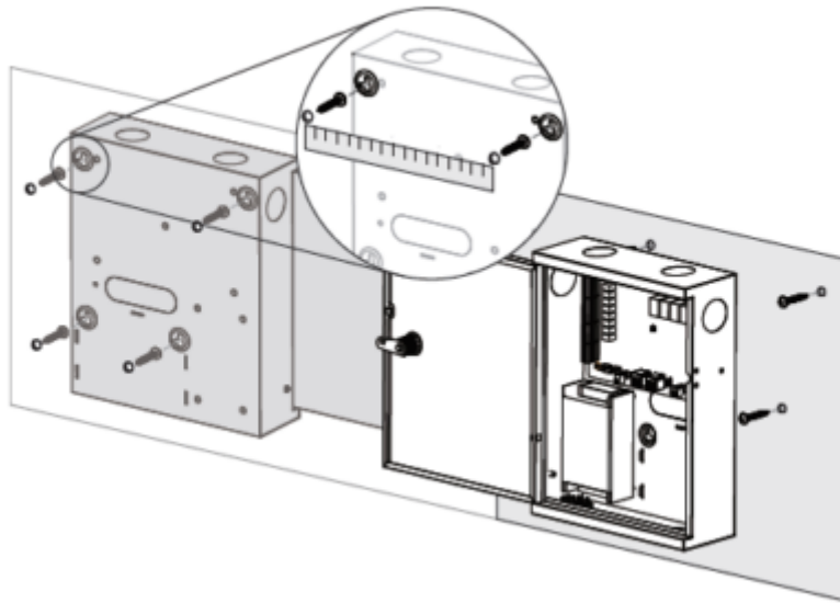
图3-3 安装示意图
