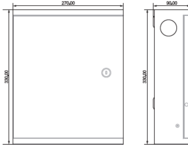
图1-1 外观尺寸
